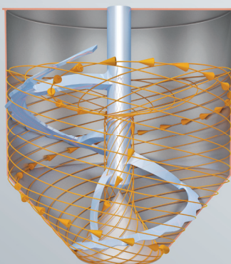
Схема движения потока продукта KoneSlid®
